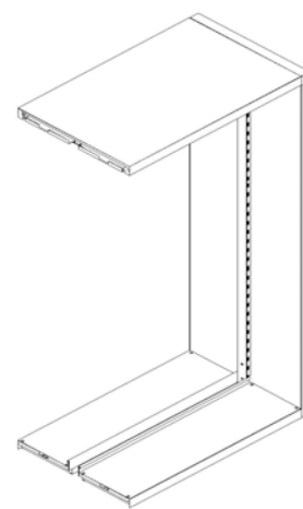
_ Detall bastiment
